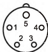
Рис. 4 Схема контактов на вилке
